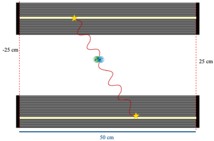
Rysunek 7.16: Schematyczny przedstawienie dwóch przeciwległych modułów wewnątrz detektora Modular J-PET, rejestrującego kwanty gamma powstające z punktu anihilacji. Tylko punkty anihilacji znajdujące się w zakresie (-25, 25) cm wzdłuż osi z są brane pod uwagę i akceptowane do dalszej analizy.
