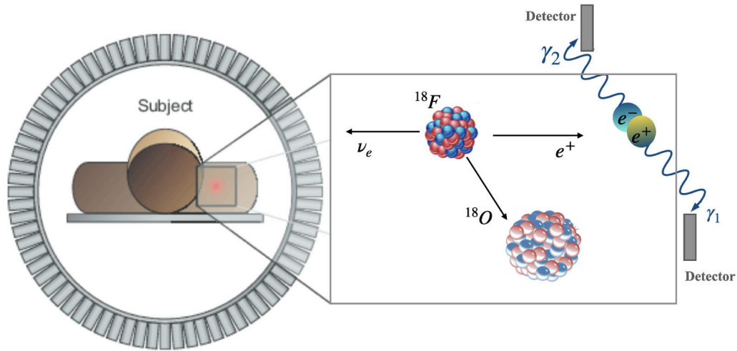
Rysunek 2.8: Schematyczny przedstawienie procesu rozpadu ^{18}\text{F} z emisją cząstki pozytonowej ( e^+ ). Emisji pozytonu towarzyszy emisja cząstki neutrino ( \nu_e ). Pozyton oddziaływa z elektronem ( e^- ) w procesie anihilacji, co prowadzi do emisji dwóch kwantów gamma o energii 511 keV. Jeden z kwantów gamma ( \gamma_1 ) jest wykrywany przez detektor, co generuje sygnał przesyłany do komputera do rekonstrukcji obrazu. Wykres oparty na [68].
